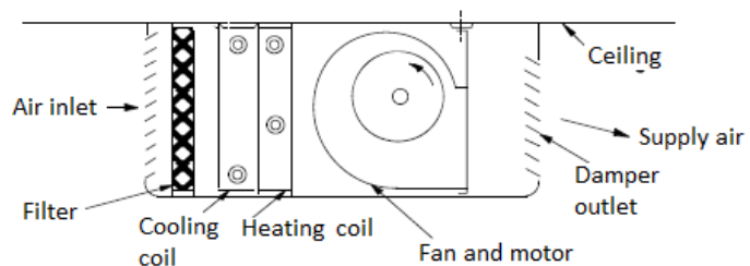
Horizontal Fan Coil Unit
